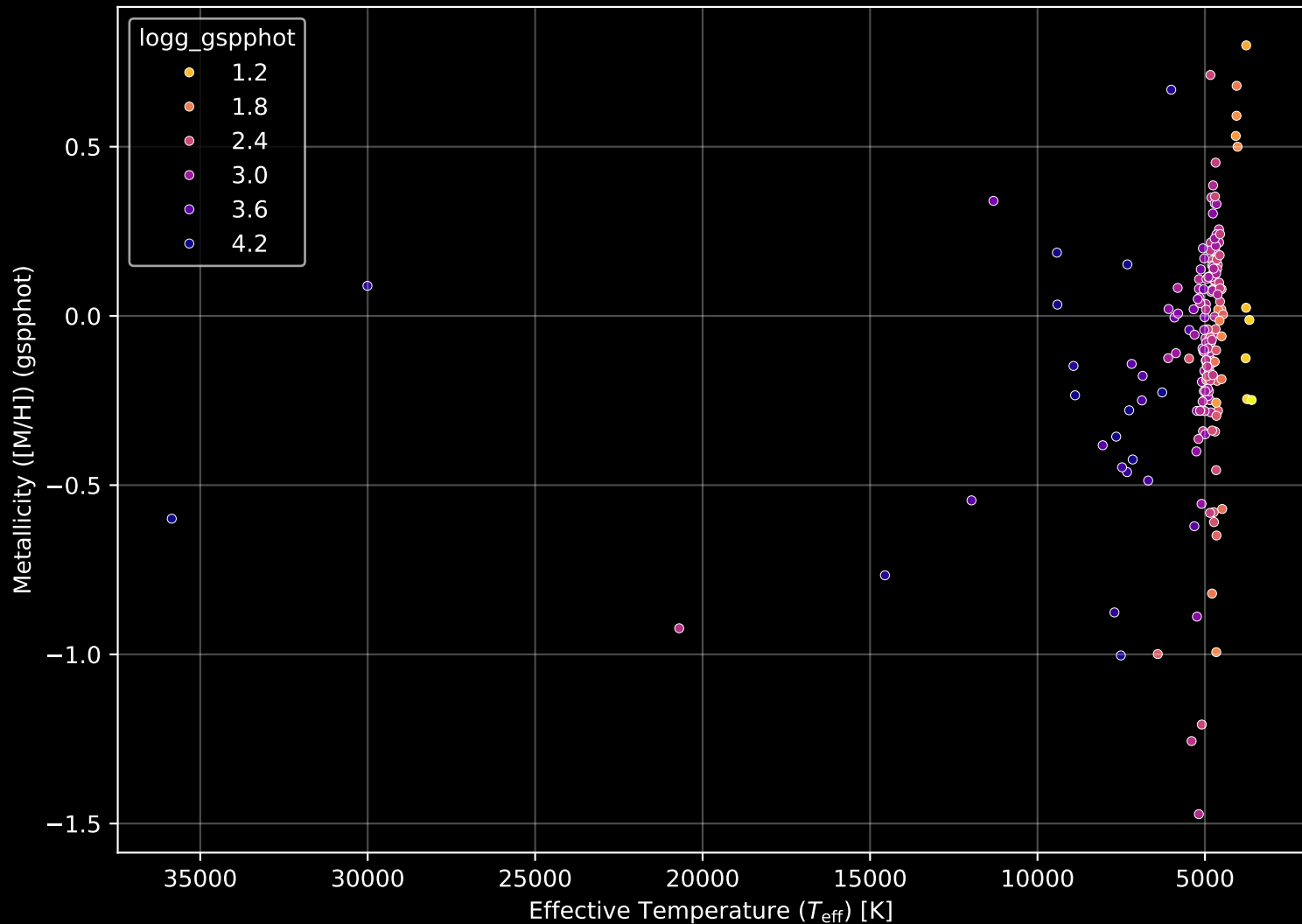
APOGEE DR17 Field: [053+04] Stellar Population Parameters (n= 189)
